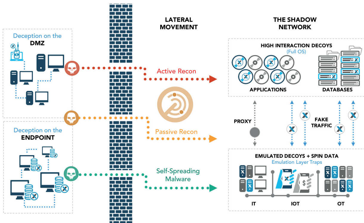
DeceptionGrid Architektur
